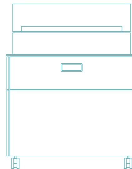
Grill Tidy Plus 943 × 1012 × 605 mm
